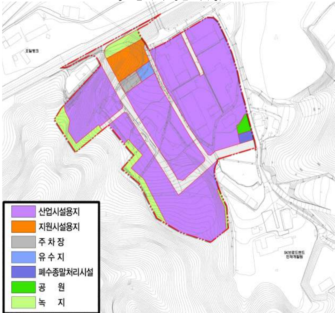
용도별 구획 평면도(기정)
